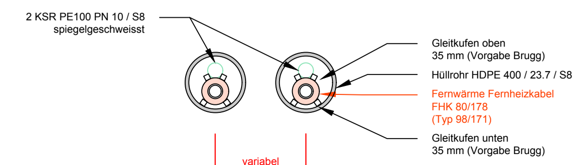
Normalprofil 1:25
